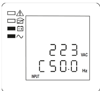
Рисунок 8 — ЖК-дисплей, Фаза С, входное напряжение и частота
