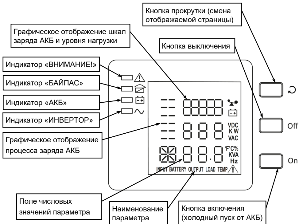
Рисунок 4 — Описание ЖК—дисплея
